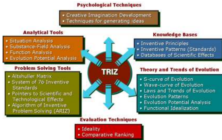
Fig 1. Modern TRIZ
